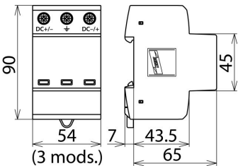
Dimensiones del DG YPV SCI 600
