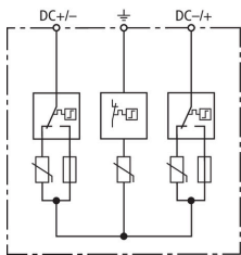
Esquema del DG YPV SCI 600
