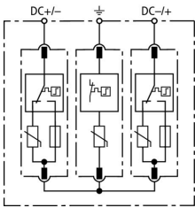
Esquema del DG M YPV SCI 150
