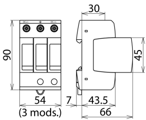
Dimensiones del DG M YPV SCI 150
