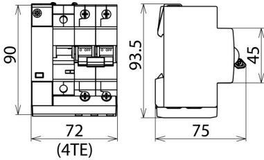
Dimensiones del SPD+POP 2 255 C40
