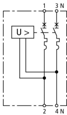
Esquema del POP 2 255 C25
