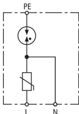
Esquema del DG TT 2P 5 275
