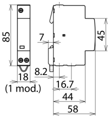
Dimensiones del DG TT 2P 5 275
