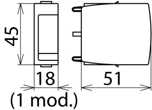
Dimensiones del DG MOD PV 500
