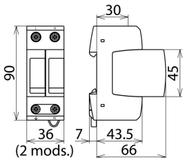
Dimensiones del DG M TT 2P 275
