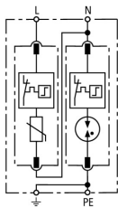
Esquema del DG M TT 2P 275
