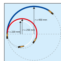
Visión global de Cable Scout+ y los radios de la torsión que ofrece.
