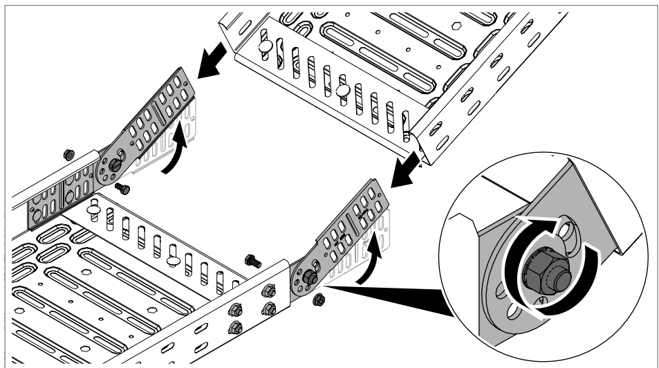
Fig. 41: Apretar el tornillo articulado
