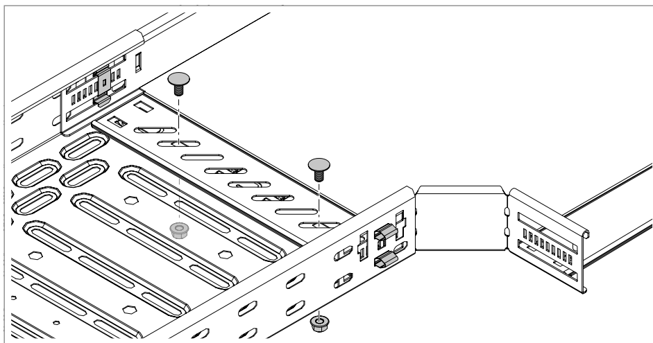
Fig. 47: Atornillar la unión recta
