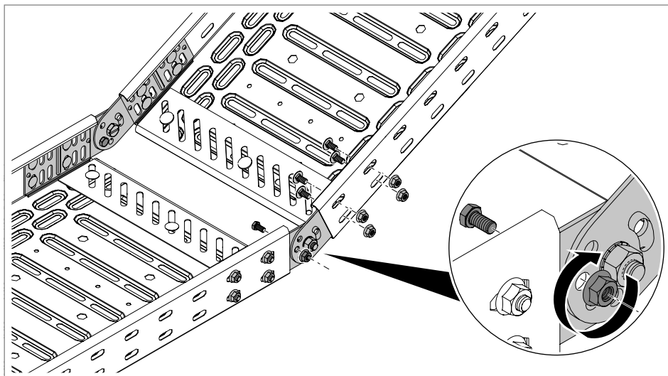
Fig. 42: Apretar el anillo de bloqueo
