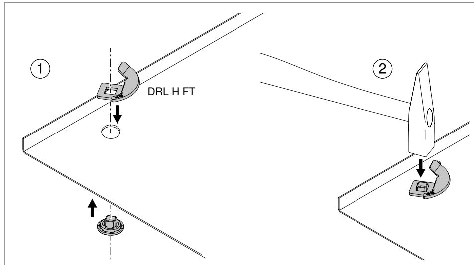
Fig. 88: Remachar el pasador giratorio
