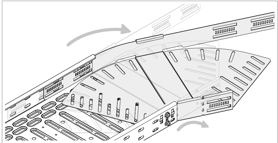
Fig. 62: Doblar la curva de ángulo ajustable
