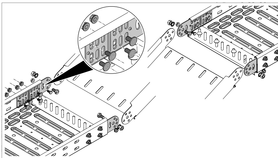
Fig. 71: Montar el conector articulado a la bandejas portacables
