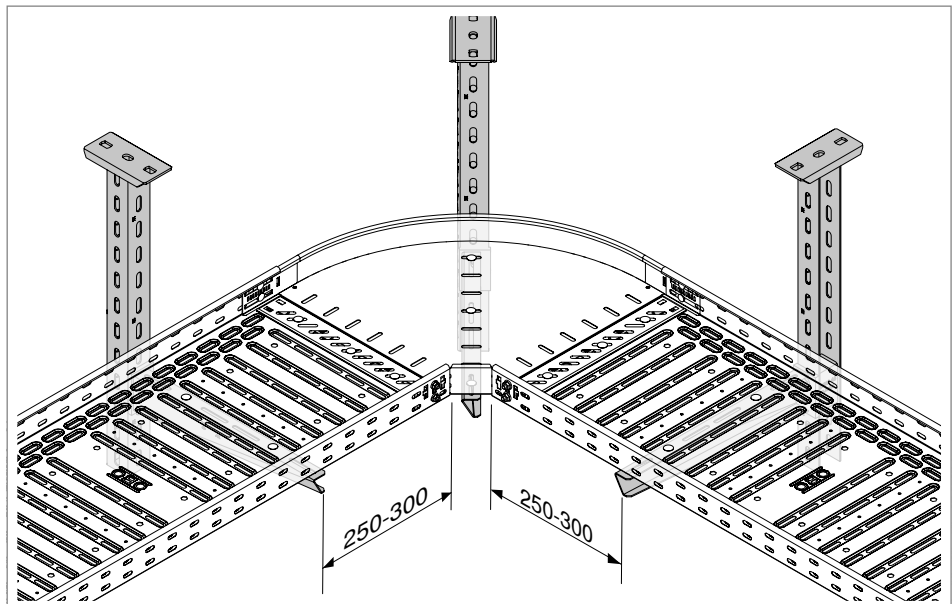
Fig. 44: Ejemplo apoyo pieza preformada curva de 90°, 400 mm de ancho
