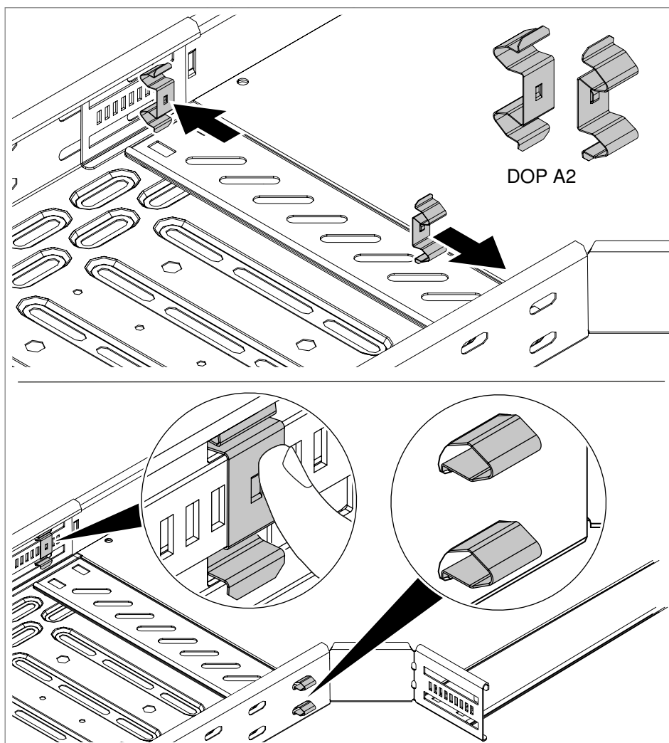
Fig. 51: Fijar la pieza preformada o accesorio con abrazadera doble
