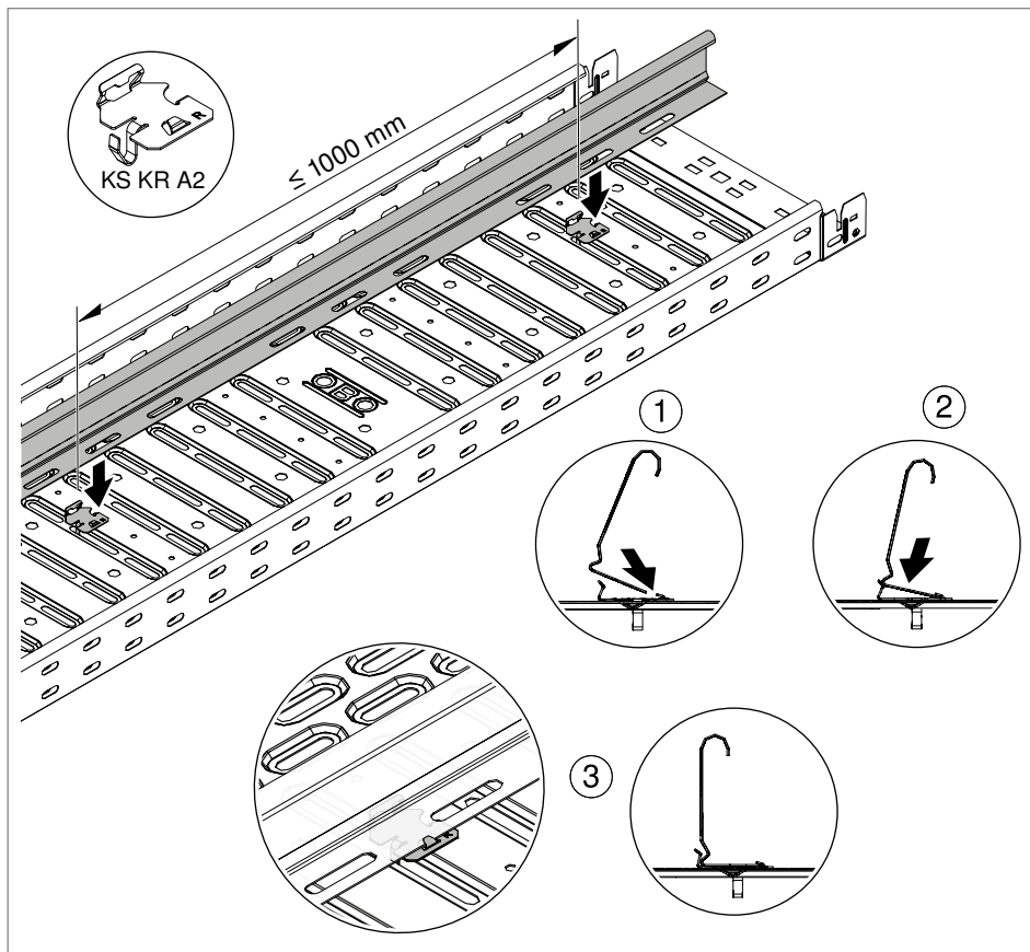
Fig. 80: Montar el tabique separador en la pieza de sujeción
