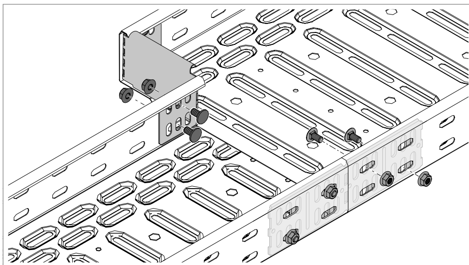
Fig. 74: Montar uniones en ángulo y rectas y reducción angular
