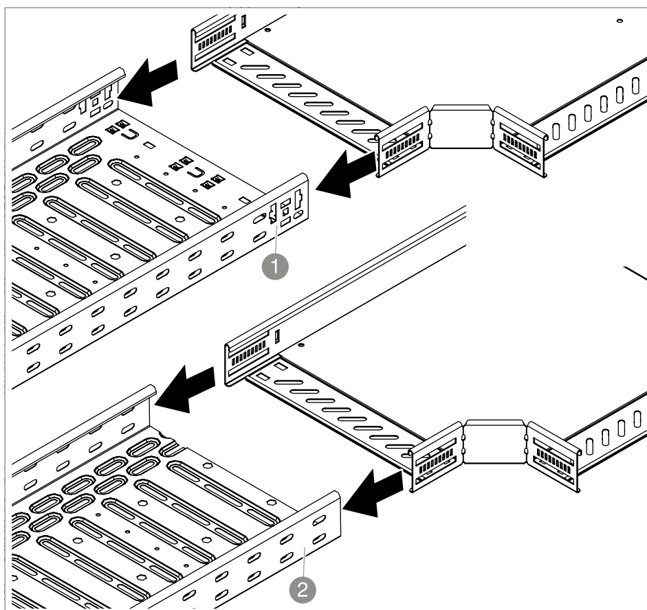
Fig. 45: Empujar la pieza preformada
