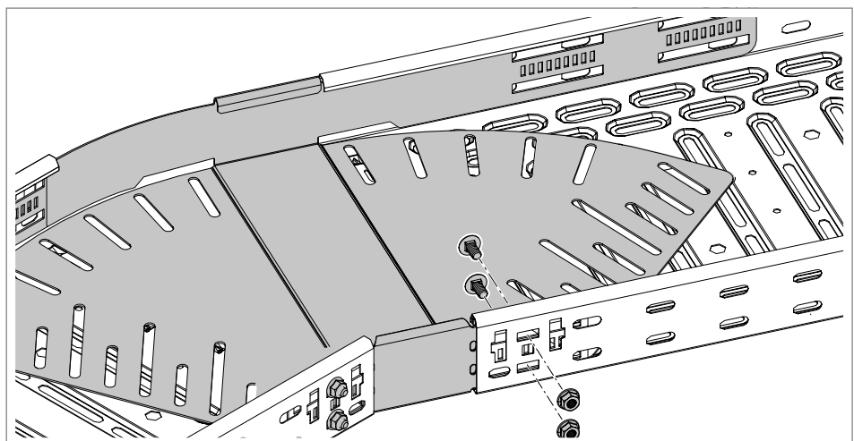
Fig. 64: Fijar la segunda bandeja a la curva
