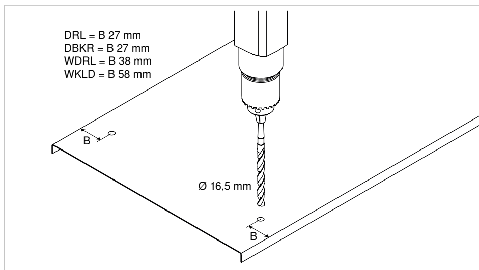
Fig. 86: Taladrar previamente la tapa
