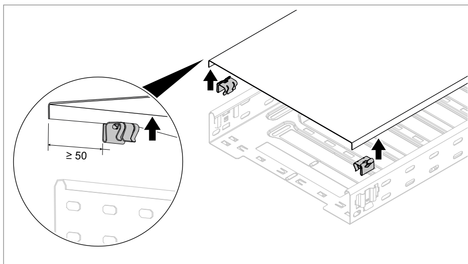
Fig. 83: Fijar la grapa específica en la tapa
