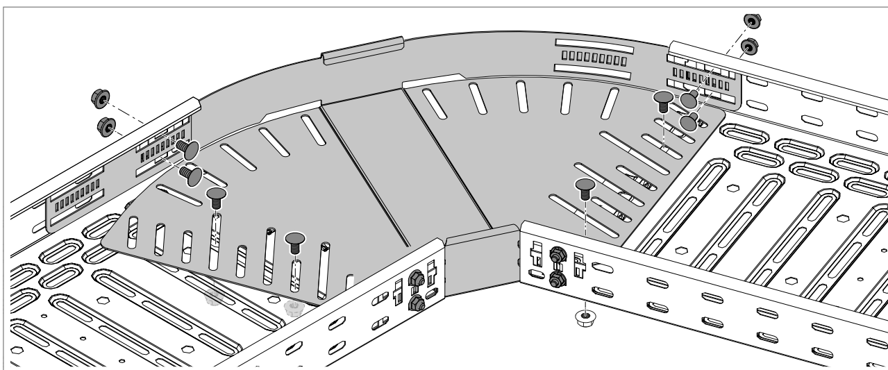
Abb. 66: Atornillar conectores y uniones a las bandejas
