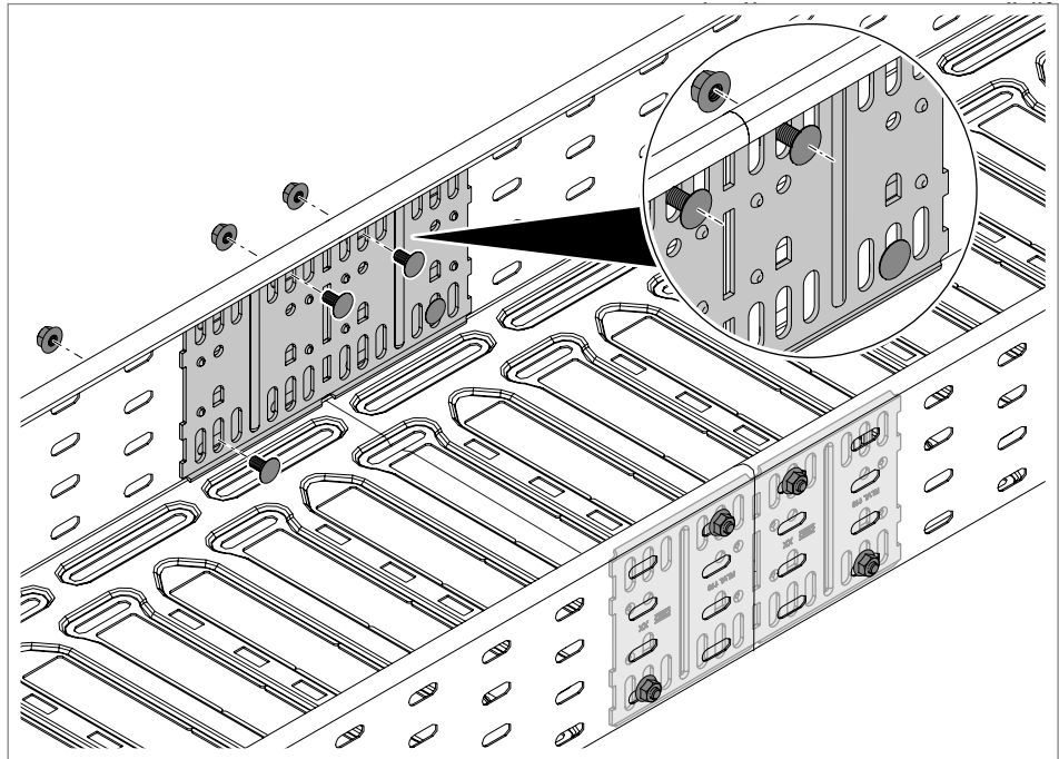
Fig. 29: Atornillar la unión recta RLVL
