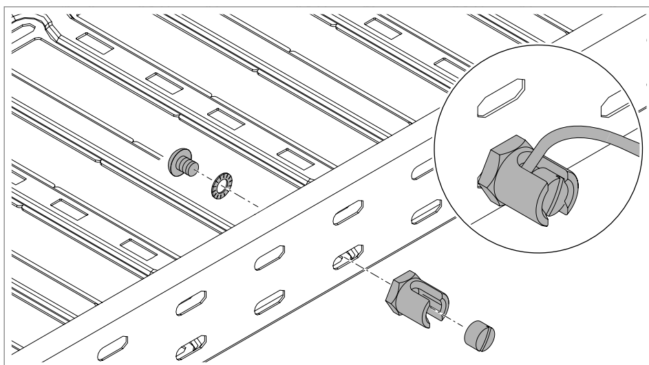
Fig. 82: Montar el borne de puesta a tierra
