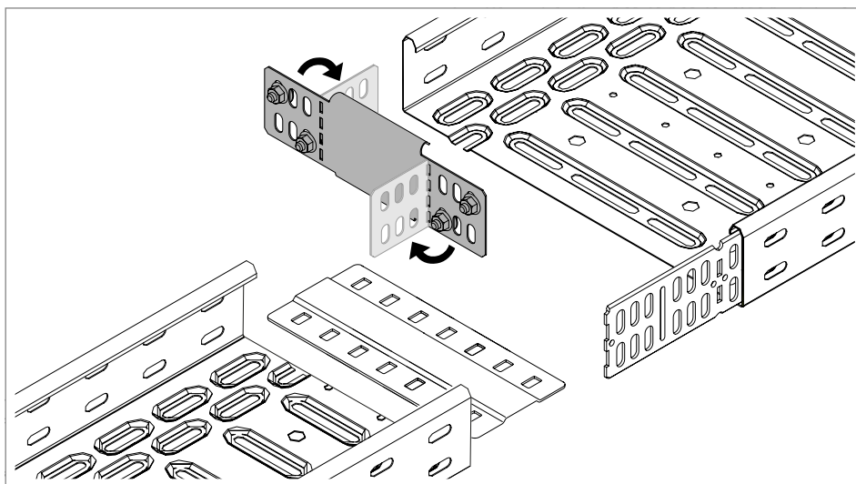
Fig. 73: Doblar reducción angular
