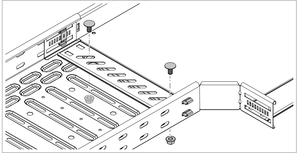
Fig. 52: Atornillar la unión recta
