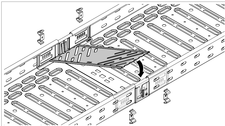
Fig. 23: Montar la unión recta de la unión recta KTSM
