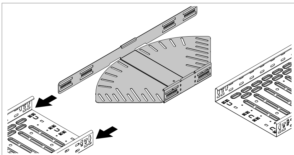
Fig. 60: Empujar la curva de ángulo ajustable
