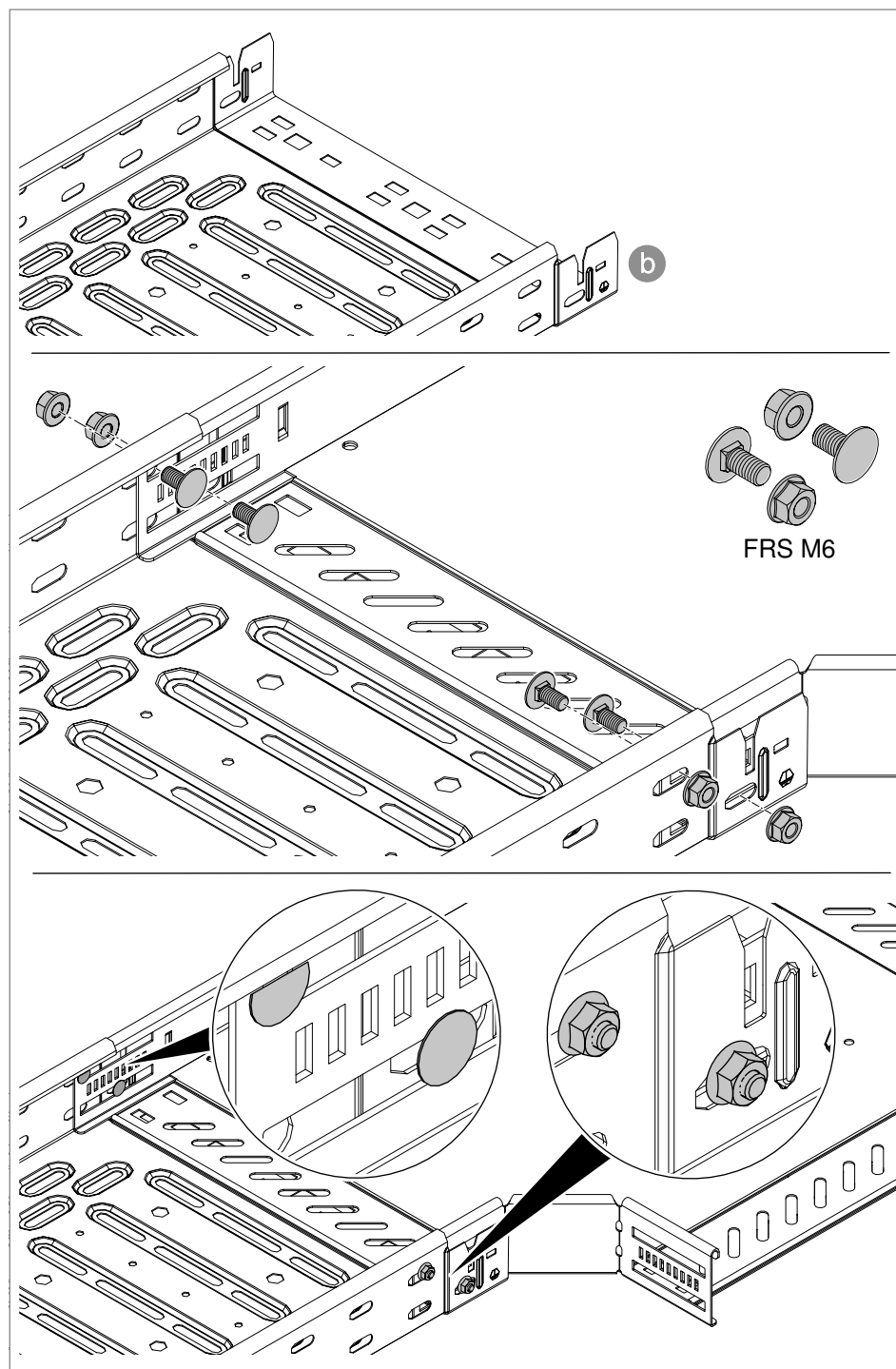
Fig. 49: Fijar la pieza preformada con tornillos (final de la bandeja b)
