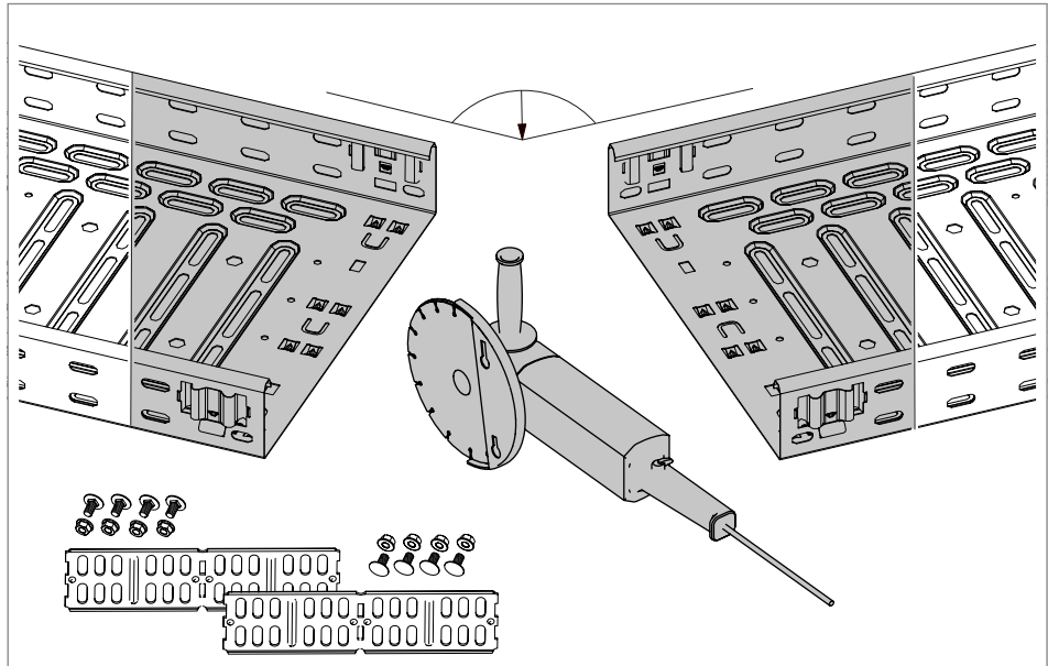
Fig. 33: Cortar la bandeja portacables para la creación de ángulo
