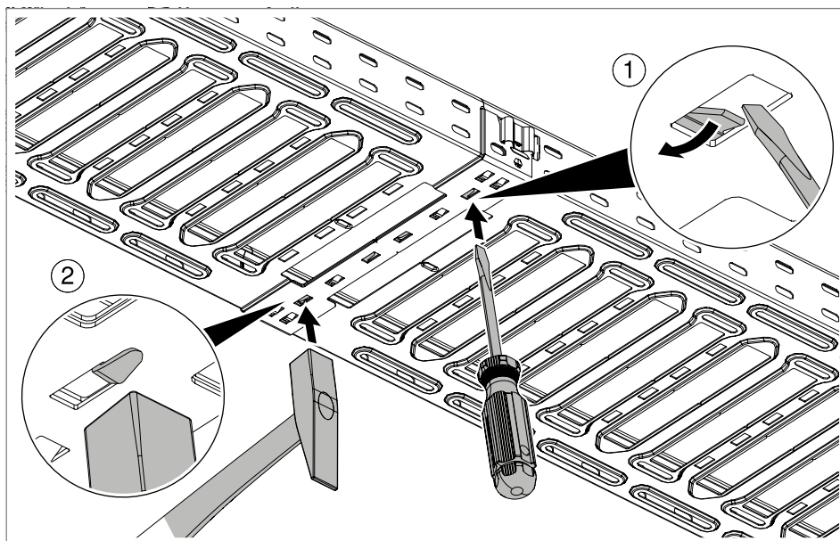
Fig. 20: Bloquear la unión de bandeja
