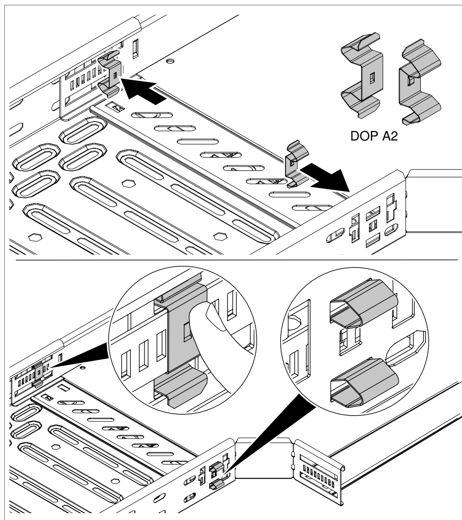
Fig. 46: Fijar la pieza preformada o accesorio con abrazadera doble
