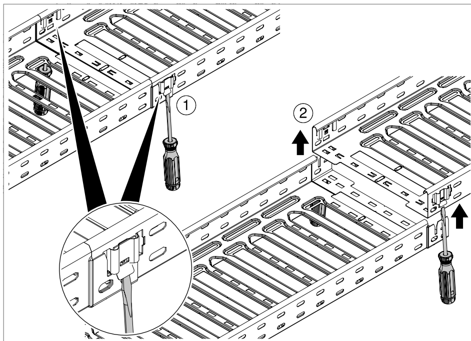
Abb. 92: Volver a soltar la unión encajable Magic
