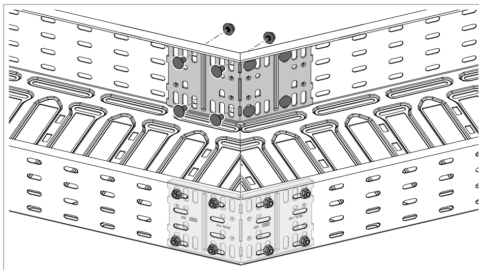
Fig. 32: Atornillar la unión recta y en ángulo RLVL
