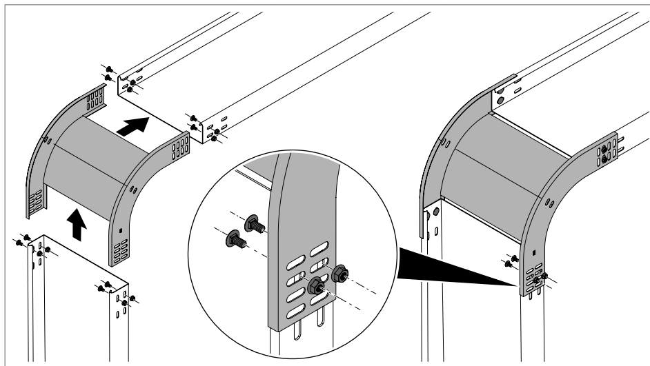
Fig. 67: Montar curva vertical descendente
