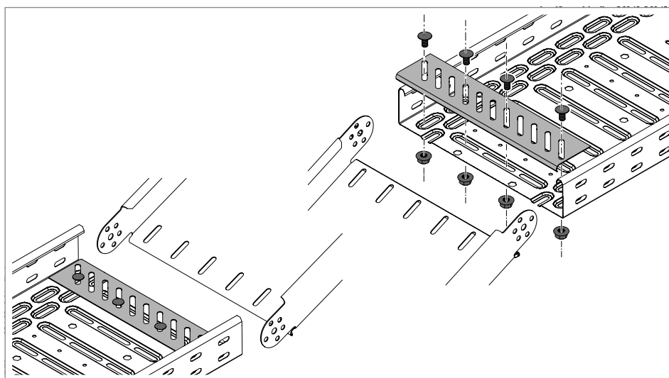
Fig. 70: Montar la chapa final de suelo
