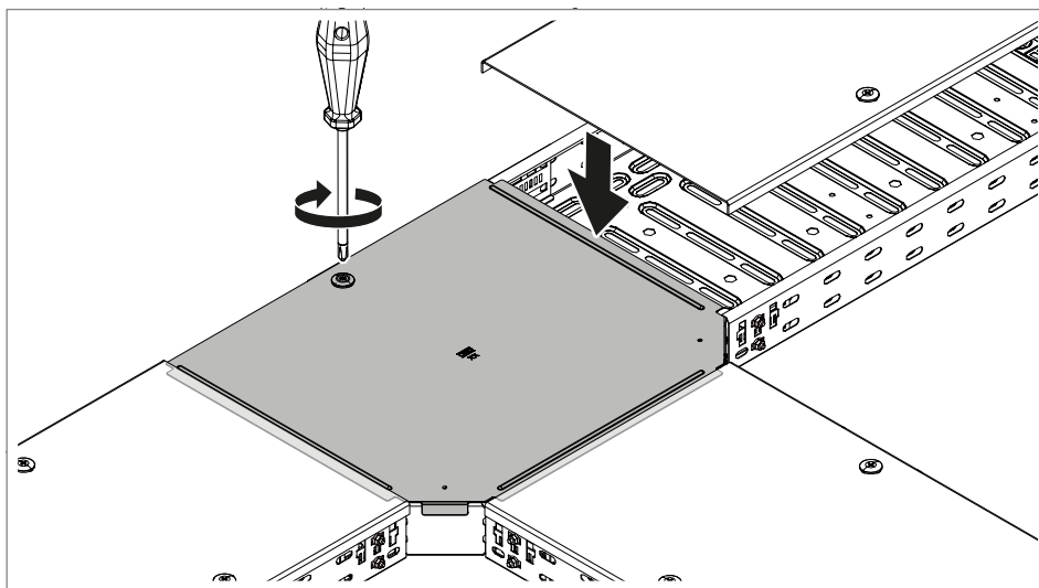
Fig. 91: Asegurar la tapa del accesorio con tapas de tramo
