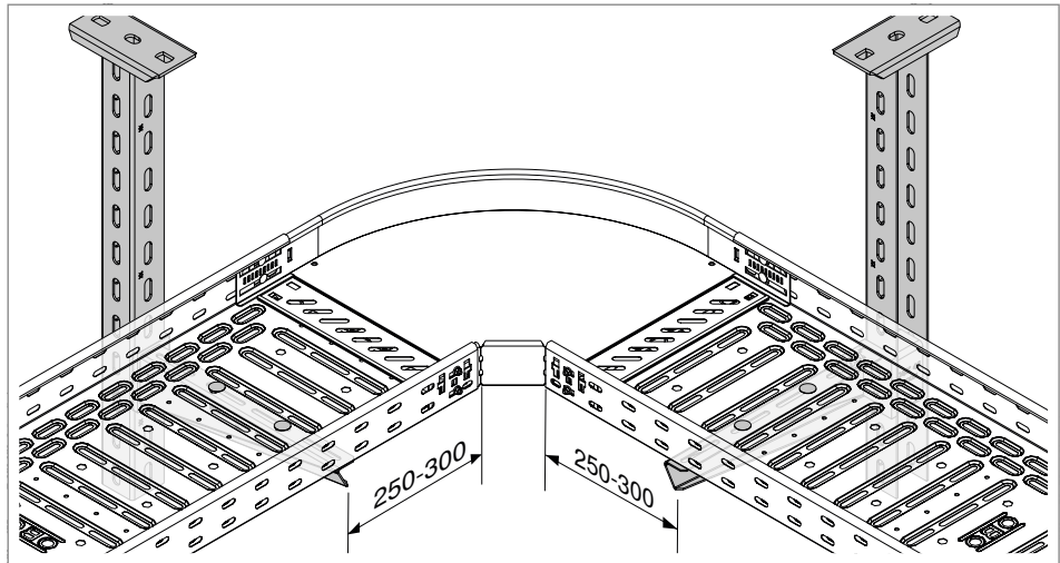
Fig. 43: Ejemplo apoyo del accesorio en curva de 90°, 300 mm de ancho
