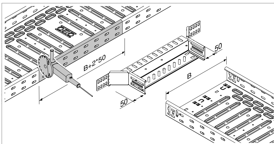
Fig. 55: Desenganchar el larguero de la bandeja portacables
