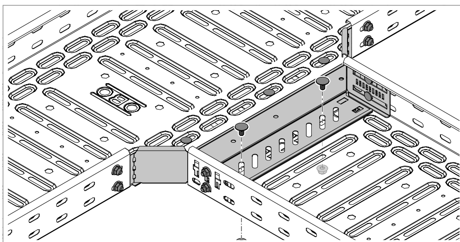
Fig. 57: Atornillar a la derivación simple la bandeja portacables que se va a desviar
