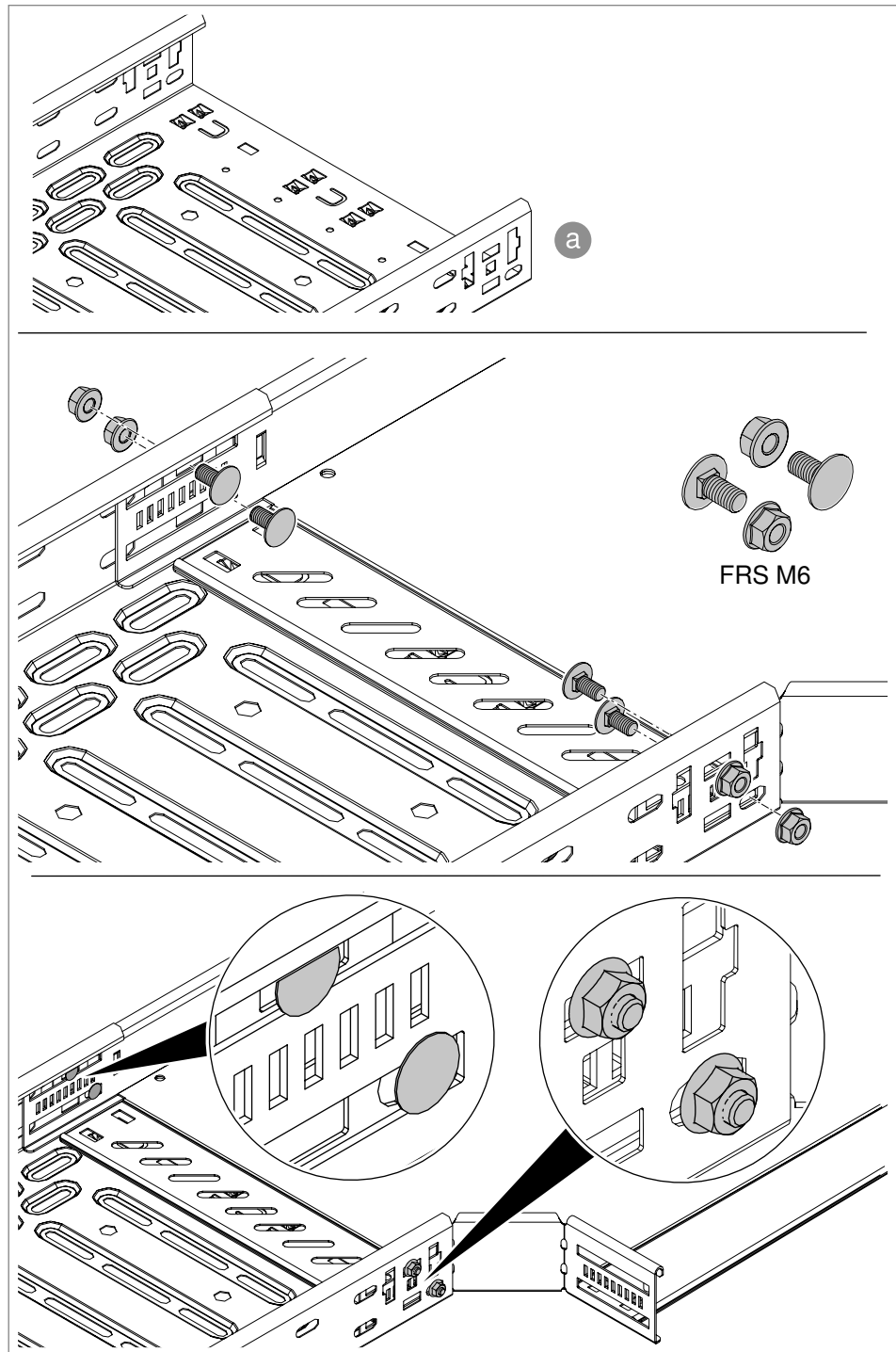
Fig. 48: Fijar la pieza preformada con tornillos (final de la bandeja (a))
