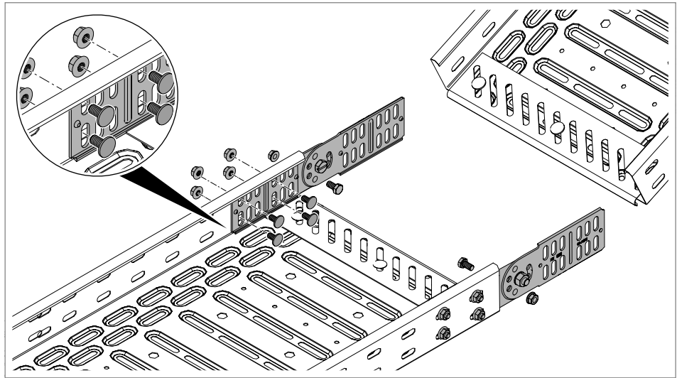
Fig. 40: Atornillar el conector articulado RGV a la bandeja portacables
