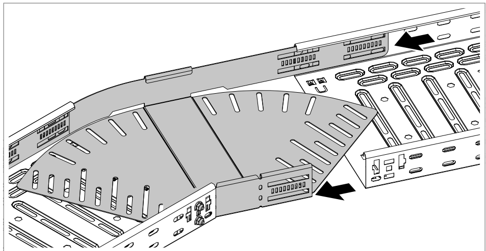
Fig. 63: Empujar la segunda bandeja hacia la curva
