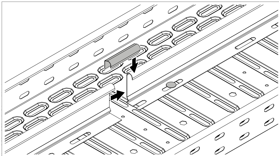
Fig. 81: Unir los tabiques separadores
