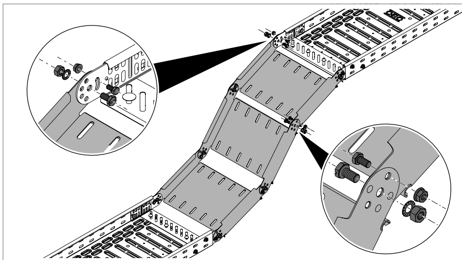
Fig. 72: Montar elementos de curva articulados
