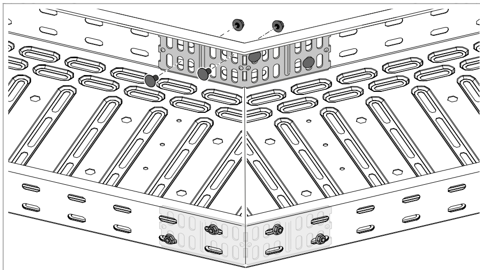
Fig. 35: Atornillar la unión en ángulo RWVL
