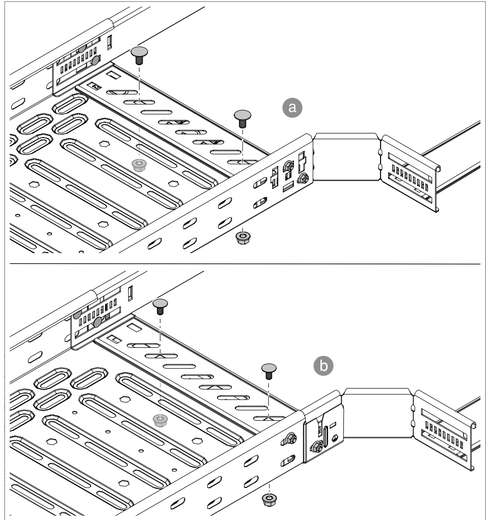
Fig. 50: Atornillar la unión recta (final de la bandeja a y b )
