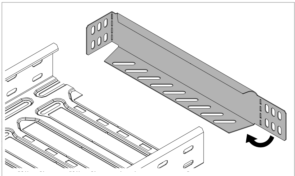
Fig. 76: Doblar la pestaña
