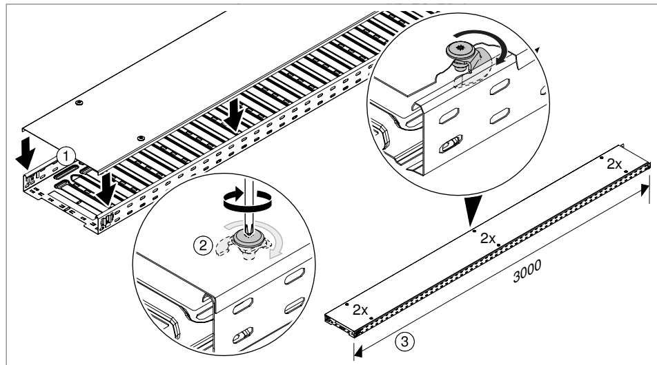
Fig. 89: Montar tapa con pasador giratorio Helix
