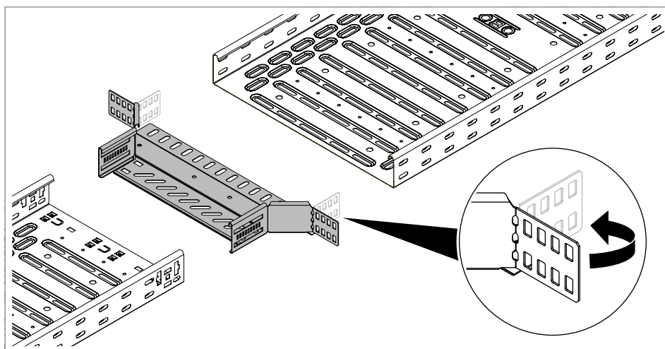
Fig. 58: Doblar la pestaña de unión
