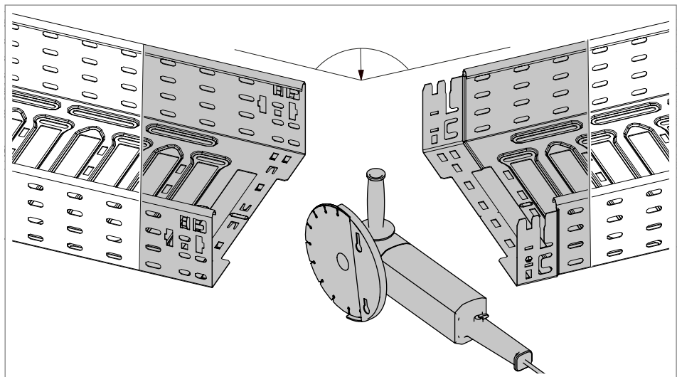
Fig. 30: Cortar la bandeja portacables para la creación de ángulo
