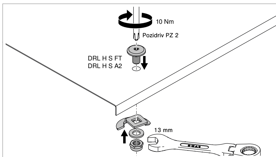
Fig. 87: Atornillar el pasador giratorio
