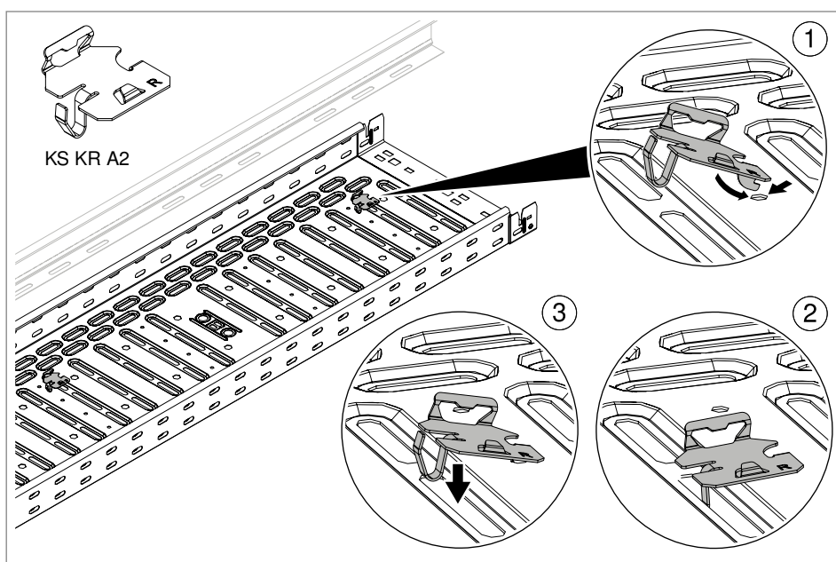
Fig. 79: Montar pieza de sujeción para tabique separador
