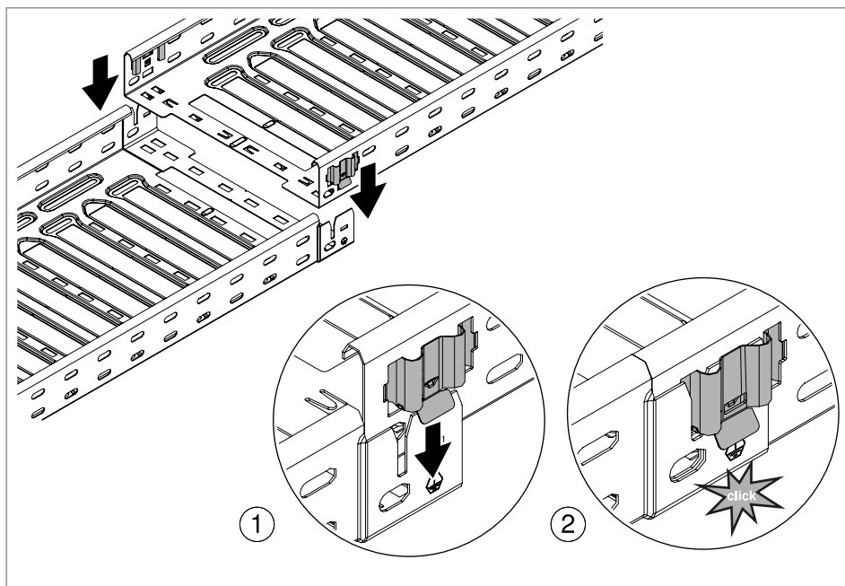
Fig. 19: Unión encajable Magic con elemento de resorte
