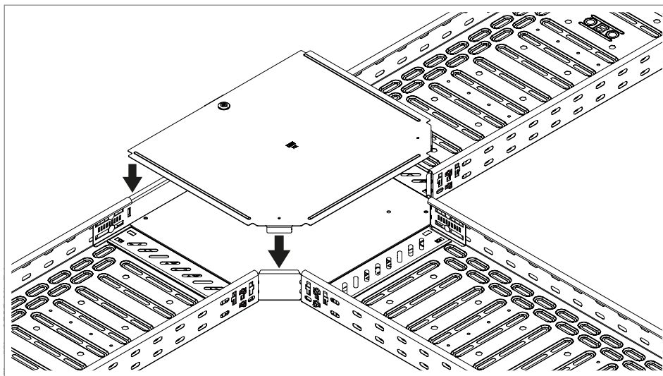
Fig. 90: Colocar la tapa del accesorio
