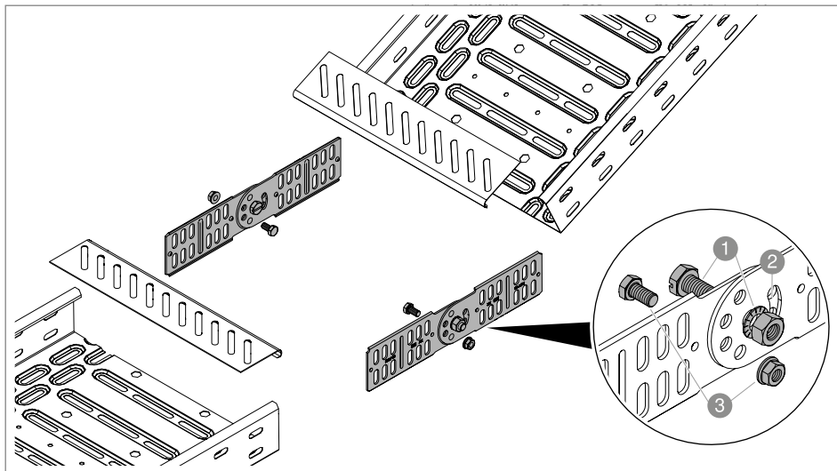
Fig. 38: Conector articulado RGV y chapas finales de suelo
