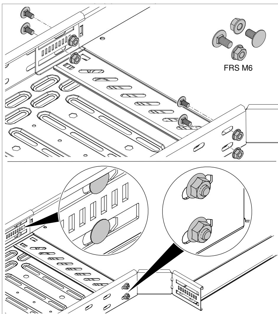
Fig. 53: Fijar la pieza preformada o accesorio con abrazadera doble
