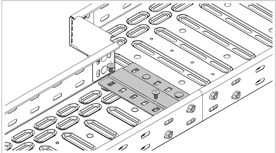
Fig. 75: Atornillar la unión recta
