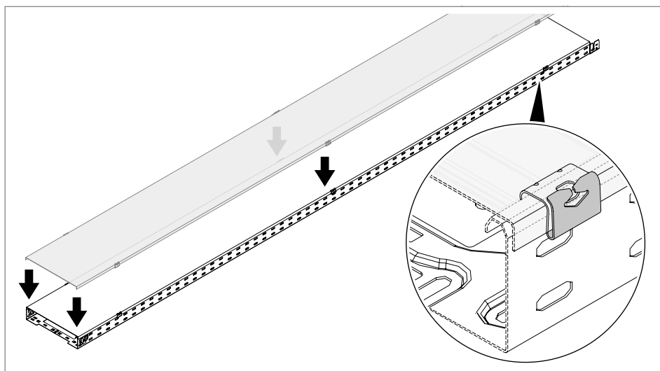
Fig. 85: Encajar la tapa
