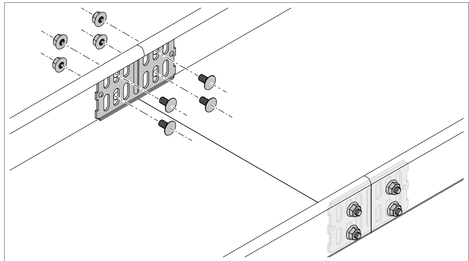
Fig. 26: Atornillar la unión recta RLVK
