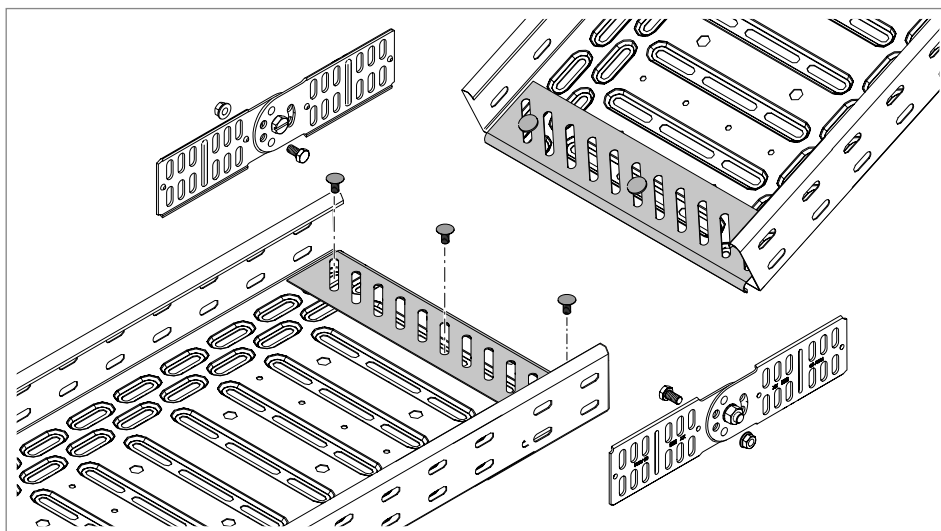
Fig. 39: Atornillar chapas finales de suelo
