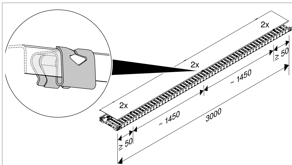
Fig. 84: Distribución del número necesario de grapas para tapa
