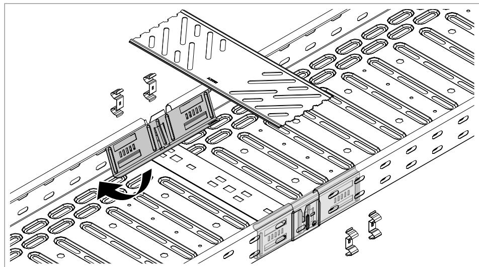
Fig. 22: Montar unión recta KTSM
