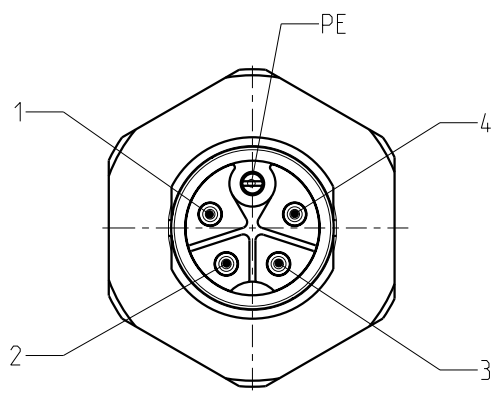
5pol K-Codierung (Steckseite) / 5pole K-coding (plug-in side)
