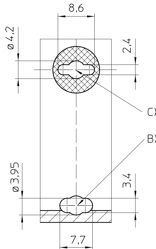
Detail1 2:1
