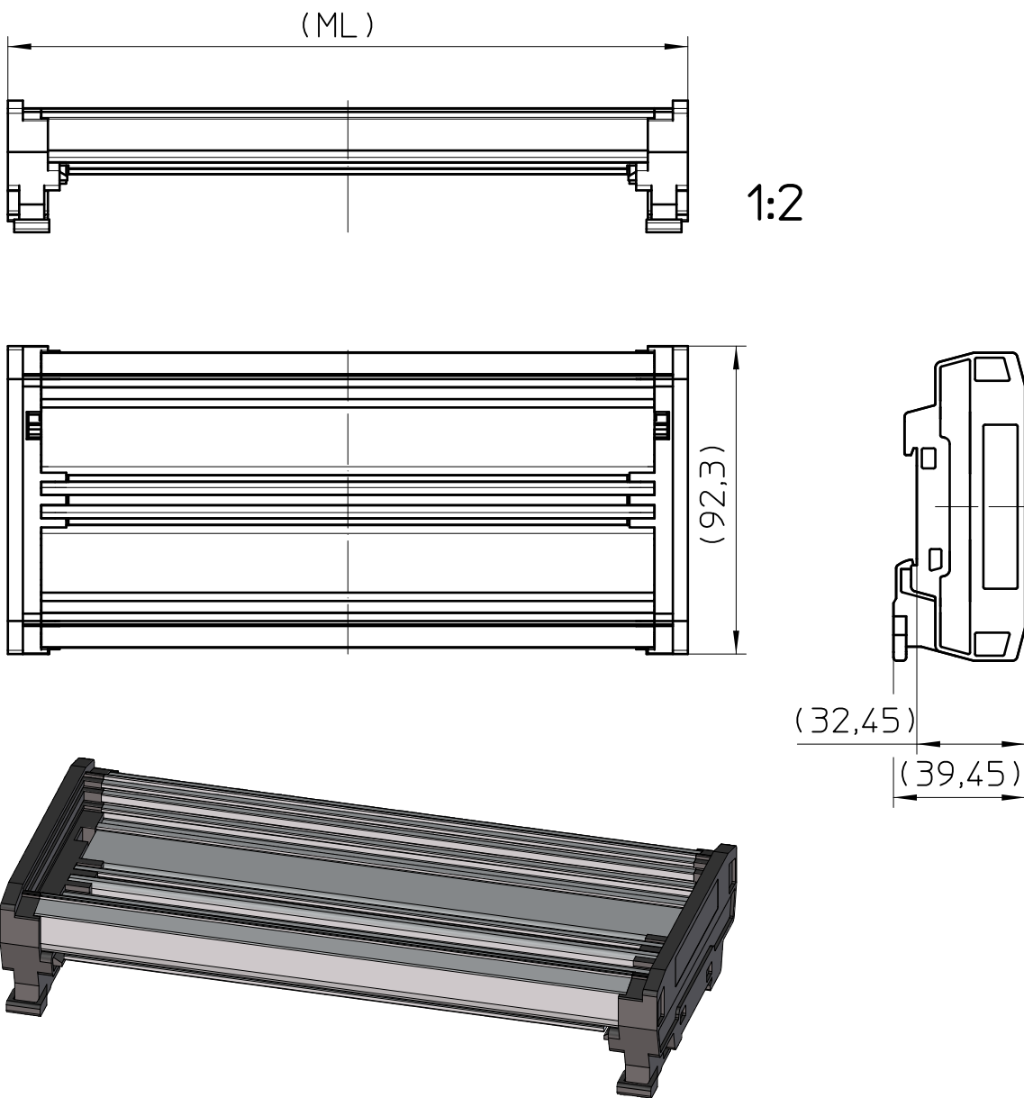
Assembly example (UM-PRO-KIT-B72-L200)
