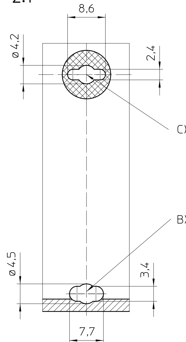
Detail1 2:1
