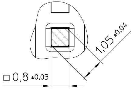
A-A 10:1
