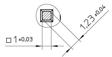
B-B 5:1
